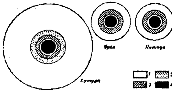
Рис.2. Внутреннее строение и предполагаемый вещественный состав некоторых планет-гигантов: 1- молекулярный водород; 2 - металлический водород; 3 - водяной лед; 4 - ядро, сложенное из каменных или железокремнистых материалов
