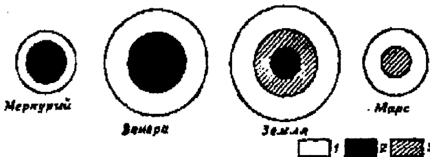
Рис.3. Структура и предполагаемый вещественный состав планет земной группы: 1- силикатное вещество; 2- металлическое; 3 - сульфид-металлическое вещество.
