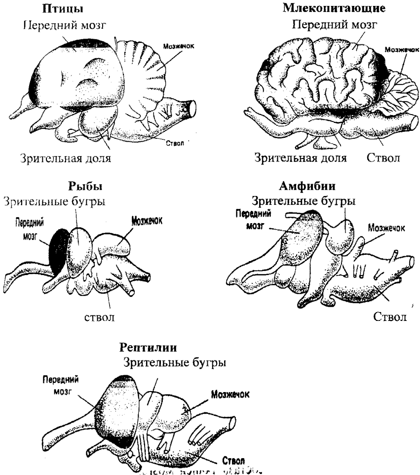
Рис. 9. Сравнение размеров основных отделов головного мозга у представителей разных групп позвоночных животных (вид сбоку). (Зрительная доля представляет собой область, связанную с восприятием света.) Обратите внимание на постепенное увеличение переднего мозга и мозжечка в ряду от рыб до птиц и млекопитающих. Передний конец мозга обращен влево.
