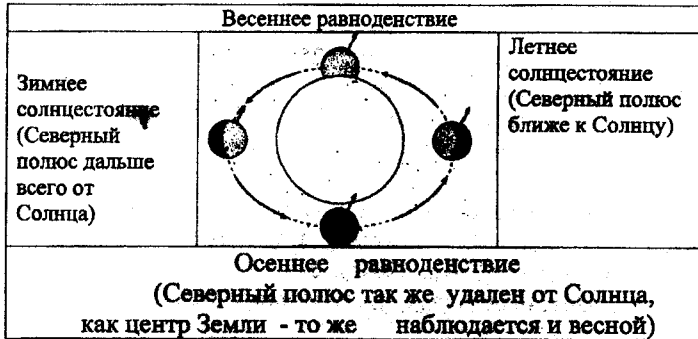
Рис. 12. Основные точки земной эклиптики
