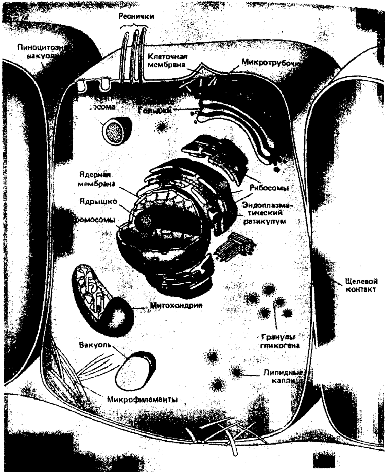
Рис. 5. Обобщенная схема клетки животного организма
