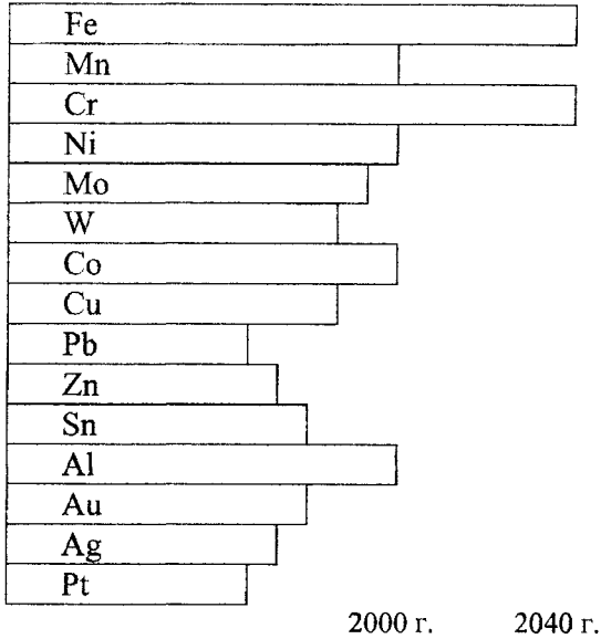
Рис. 11. Мировые запасы некоторых металлов
