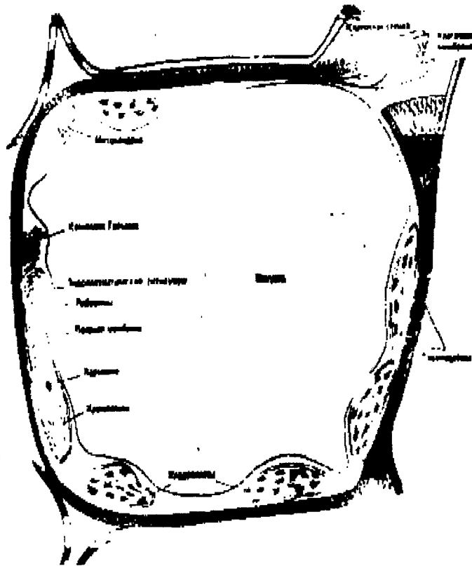
Рис.6. Обобщенная растительная клетка
