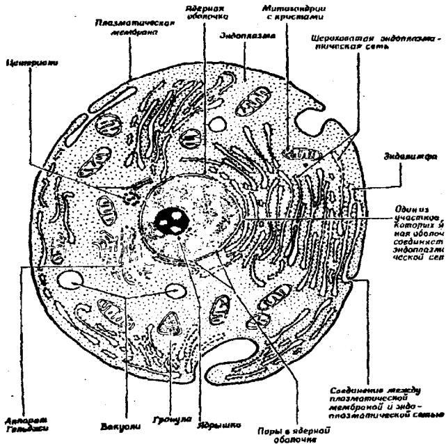
Рис. 4. Современная схема строения эукариотической живой клетки. Видно расположение различных клеточных компонентов
