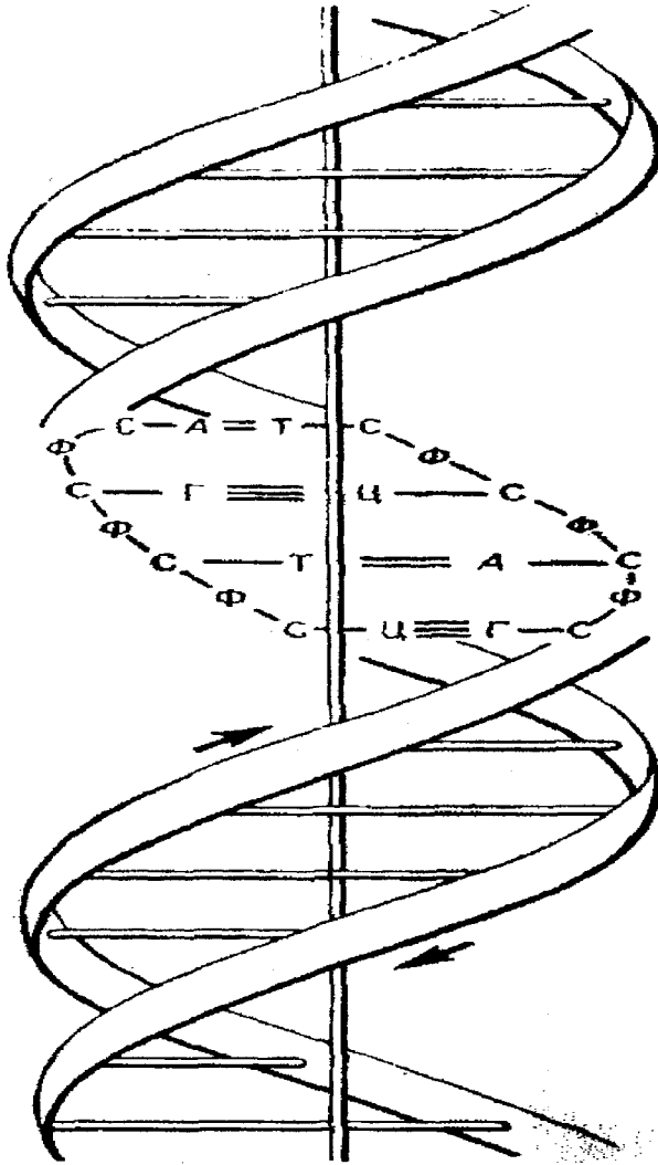
Рис.7.Схема строения важнейшего биополимера дезоксирибонуклеиновой кислоты (ДНК). Молекула ДНК представляет собой двойную спираль; буквами обозначены входящие в нее нуклеотиды
